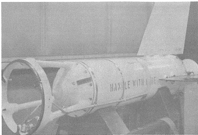
(d) Booster motor.
