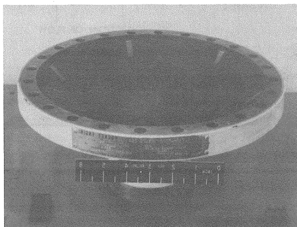
(d) Side view of nozzle closure.
